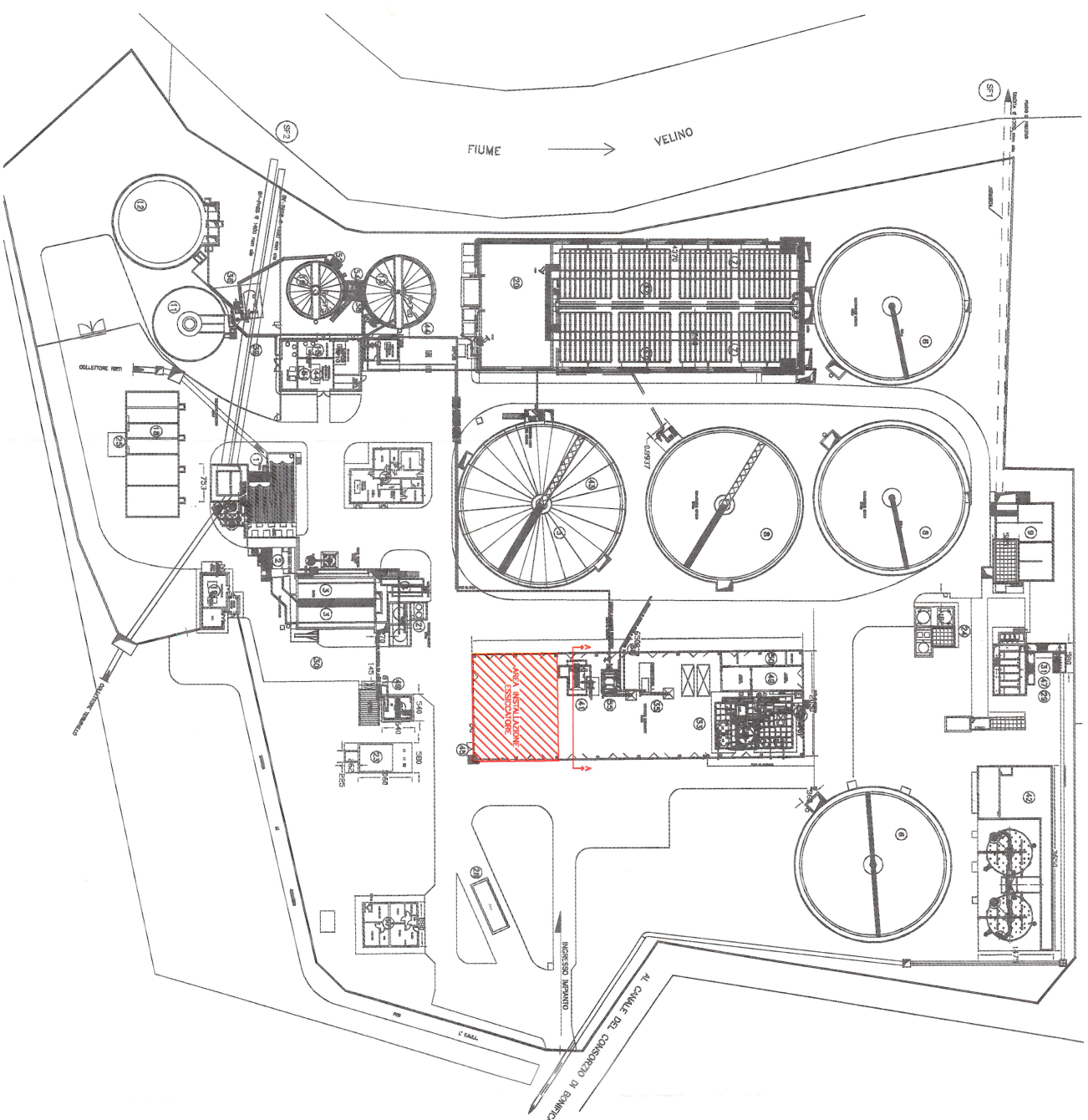
PLANIMETRIA GENERALE IMPIANTO DI DEPURAZIONE SCALA 1:500
